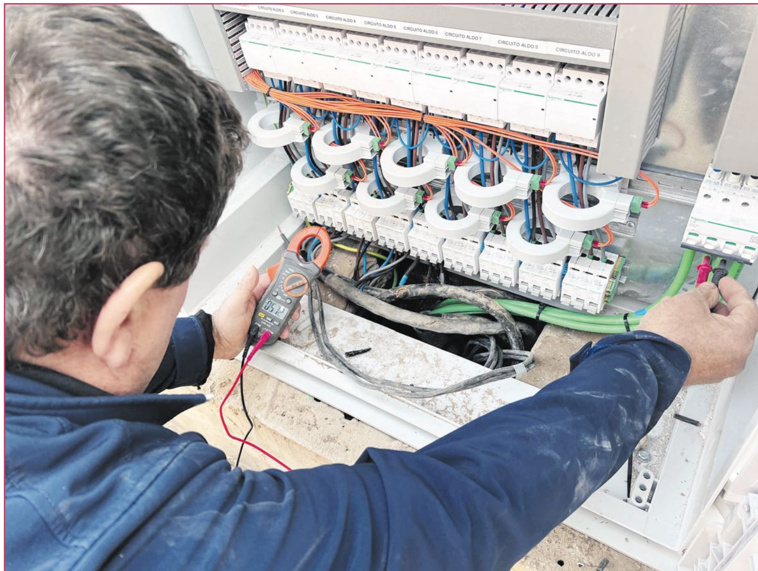
Instalación de un nuevo cuadro eléctrico.
